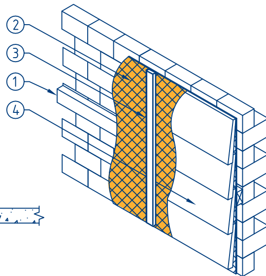
DETAIL 2 SCALE: 1:25
